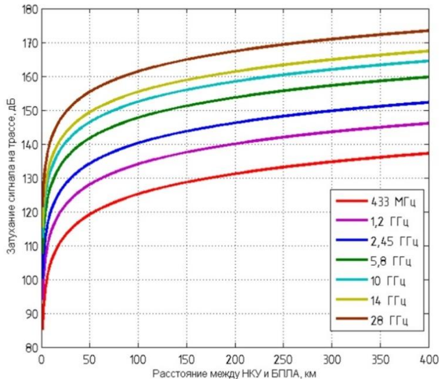
Рис. 1. Затухание радиосигнала различных диапазонов волн при распространении в атмосфере в зависимости от дальности 4 .
