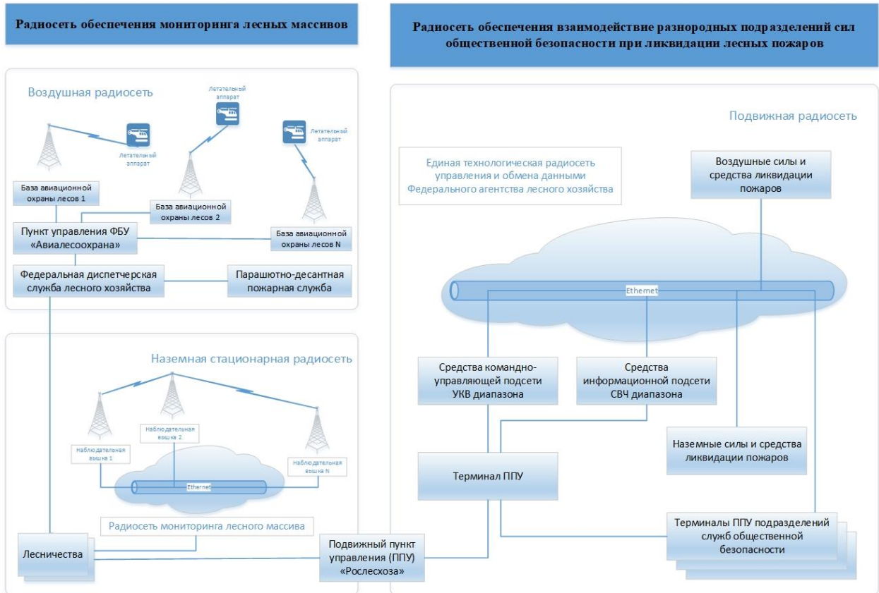
Рис. 1. Общая схема радиосети обмена данными, позволяющей обеспечить взаимодействие подразделений служб общественной безопасности при проведении совместных операций по ликвидации лесных пожаров.
