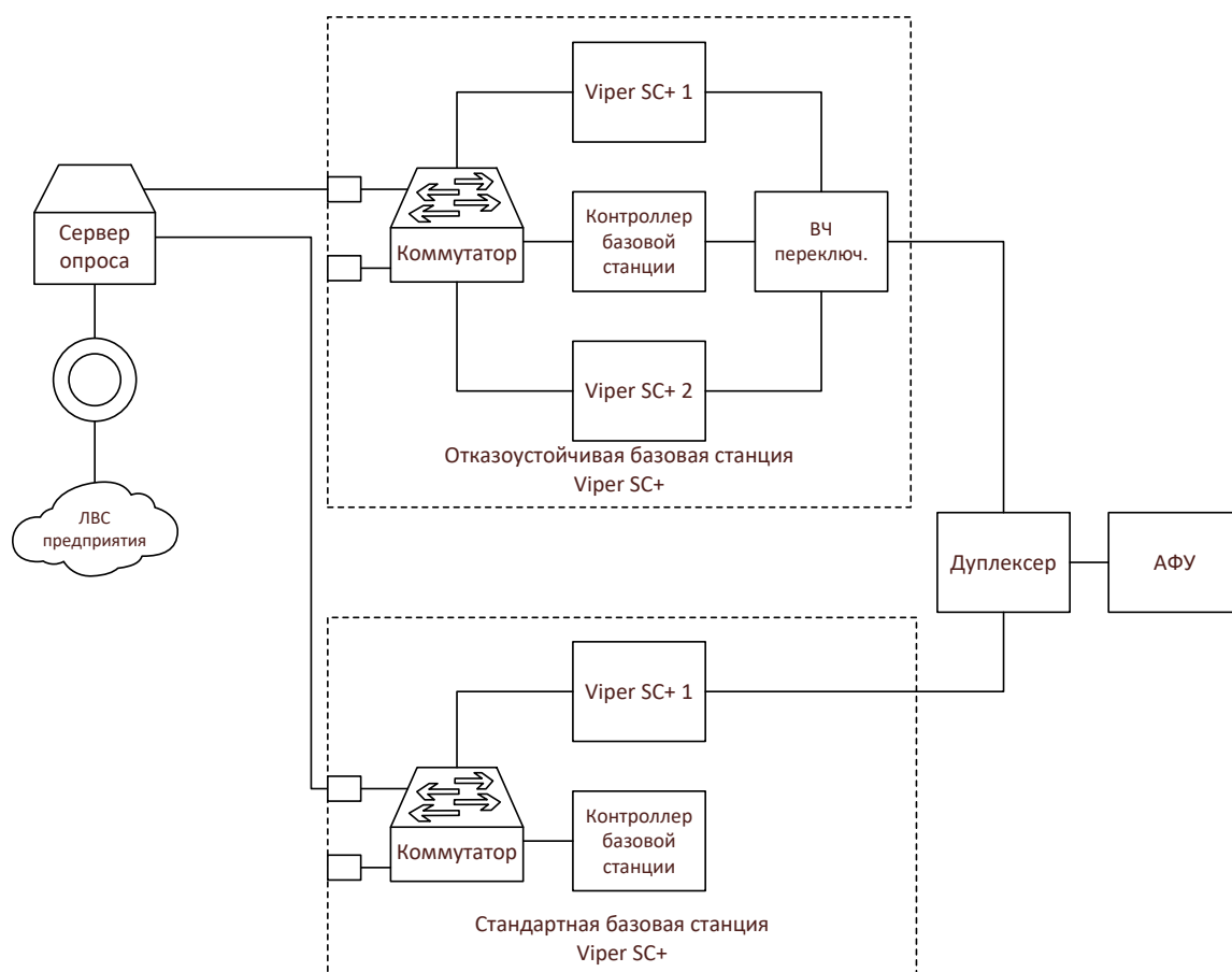
Рис. 2. Структурная схема базовой станции повышенной надежности и живучести, имеющей в своем составе: а) два комплекта оборудования Viper-SC+ base station (140-5118-502); б) комплект оборудования Viper-SC+ base station (140-5318-502) с дублированием приемопередатчиков и Viper-SC+ base station (140-5118-502).
