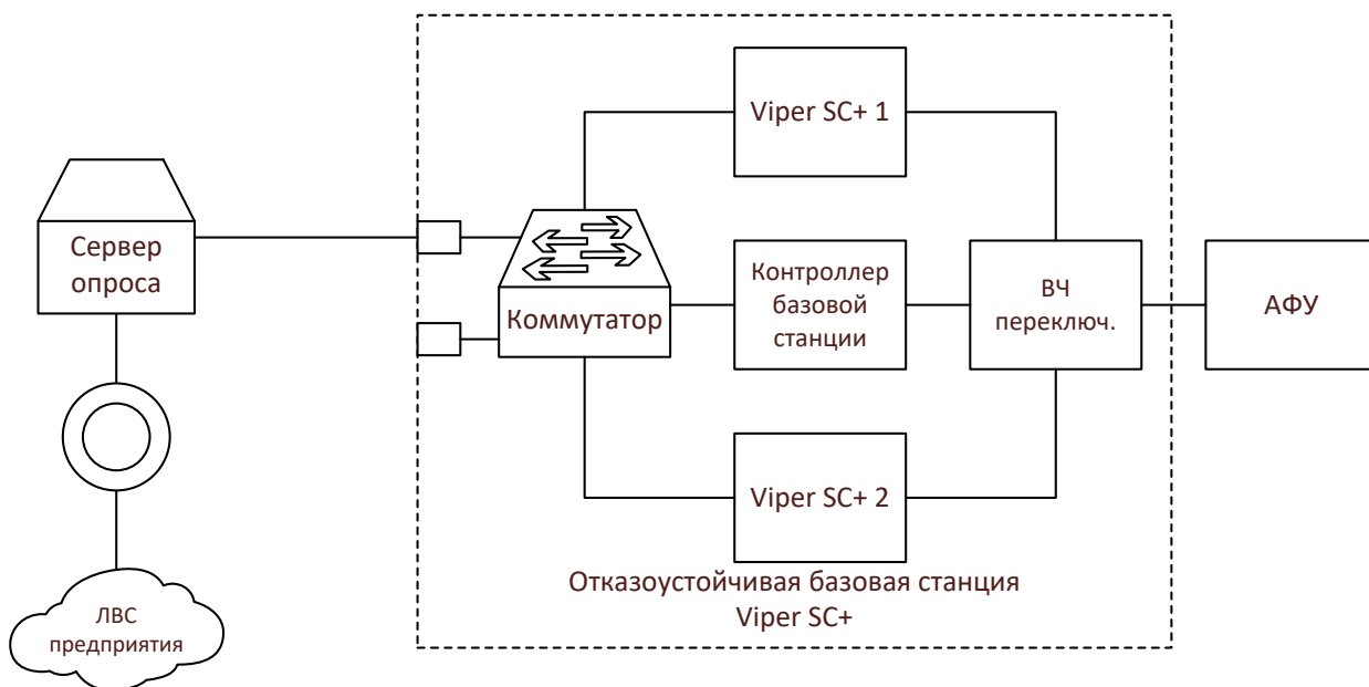
Рис. 1. Структурная схема базовой станции повышенной надежности и живучести на оборудовании Viper-SC+ base station (140-5318-502).
