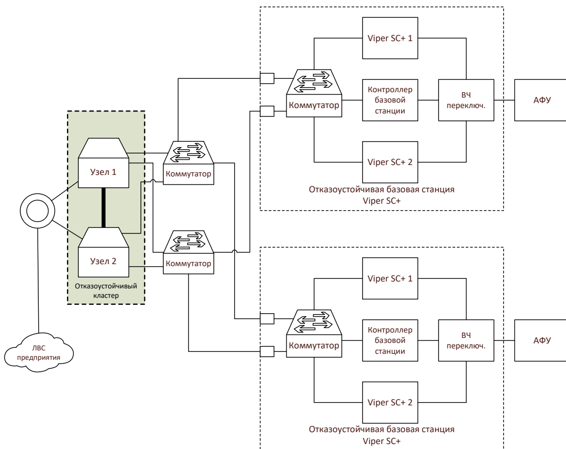
Рис. 10. Структурная схема базовой станции повышенной надежности и живучести на оборудовании Viper-SC+ base station (140-5318-502) с подключением к серверу третьего уровня отказоустойчивости и не имеющей единой точки отказа с двумя антенно-фидерными устройствами.
