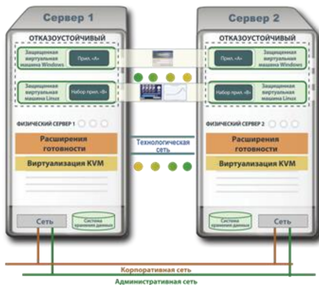
Рис. 5. Упрощенная схема вычислительного комплекса повышенной надежности и живучести под управлением ПО Stratus everRun.
