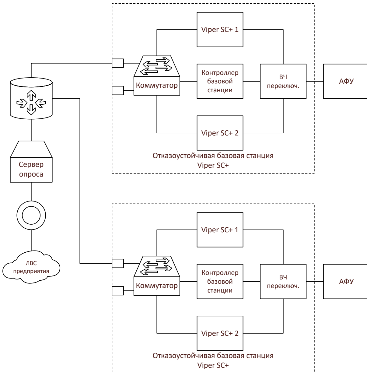
Рис. 4. Структурная схема базовой станции повышенной надежности и живучести, имеющей в своем составе два комплекта оборудования Viper-SC+ base station (140-5318-502), с двумя антенно-фидерными устройствами.
