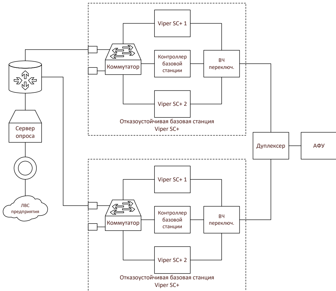
Рис. 3. Структурная схема базовой станции повышенной надежности и живучести, имеющей в своем составе: а) два комплекта оборудования Viper-SC+ base station (140-5118-502); б) Viper-SC+ base station (140-5318-502) с дублированием приемопередатчиков.
