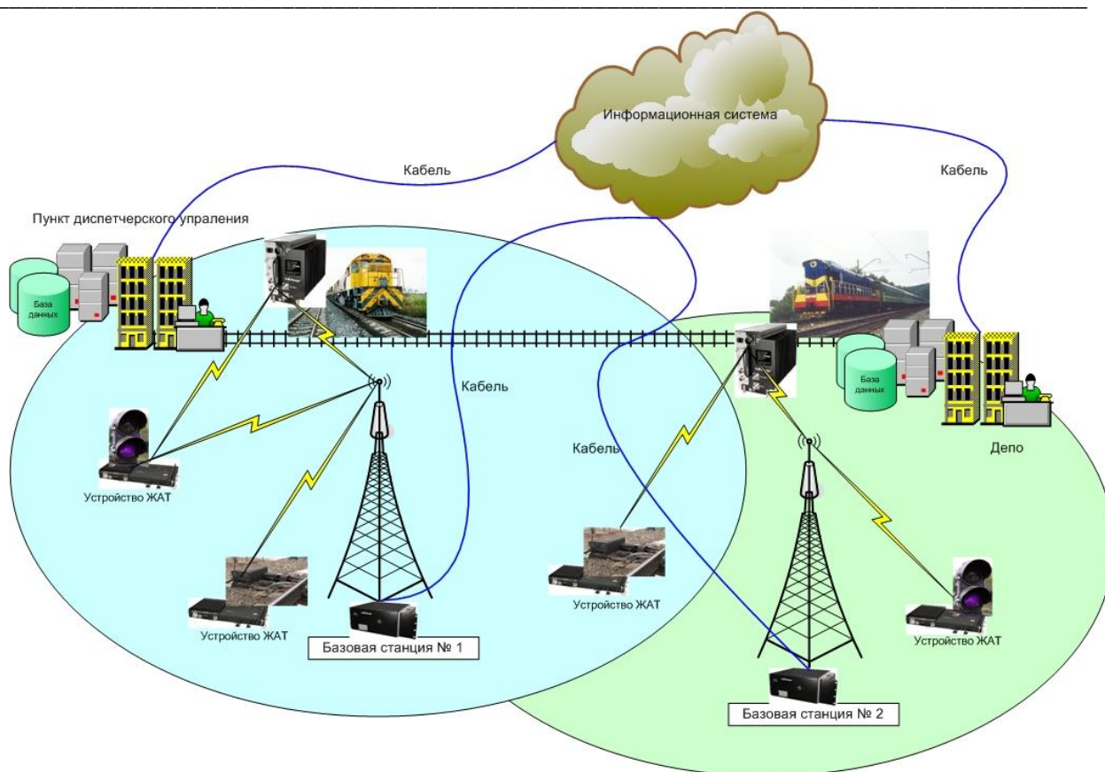
Рис. 4. Упрощенная схема технологической радиосети обмена данными для перспективной автоматизированной системы управления поездами на базе радиотехнической платформы ИТС 220.
